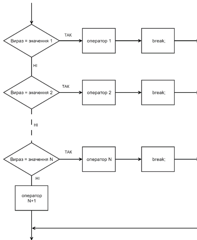
Рисунок 8 - Алгоритми роботи оператора switch/case
