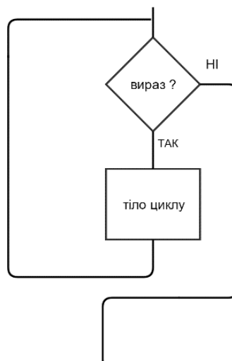
Рисунок 9 – Цикл while
