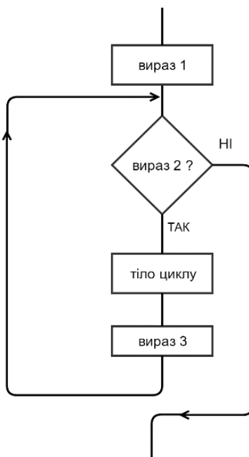
Рисунок 10 – Цикл for
