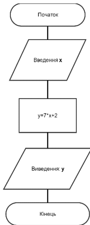
Рисунок 6 - Лінійний алгоритм
